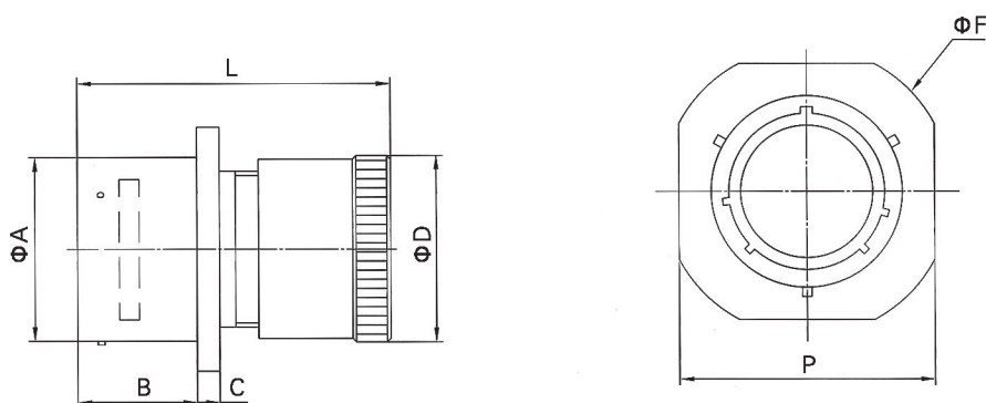
电缆连接插座 (E类)
