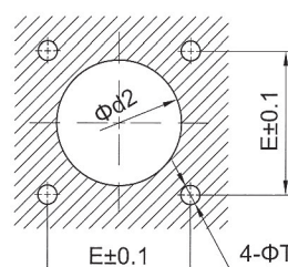
推荐面板开孔尺寸
