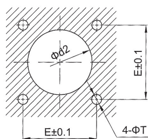
推荐面板开孔尺寸
