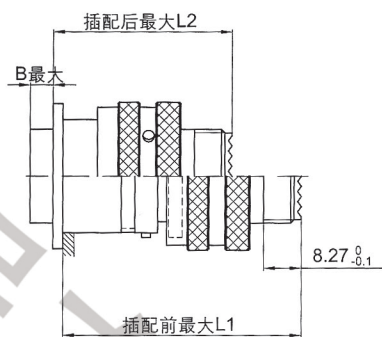
盒式方盘后装 插座 ( JY27505 ) / 插头 ( JY27467 )
