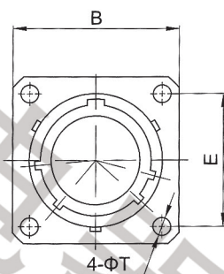
推荐面板开孔尺寸
