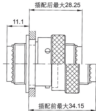
墙式方盘后装 插座 ( JY27497 ) / 插头 ( JY27473 )
