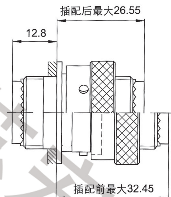
盒式方盘前装 插座 ( JY27513 ) / 插头 ( JY27473 )
