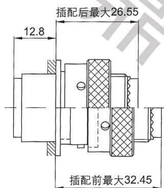
盒式方盘前装 插座 ( JY27513 ) / 插头 ( JY27473 )
