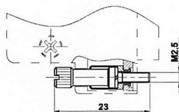
外形尺寸图
