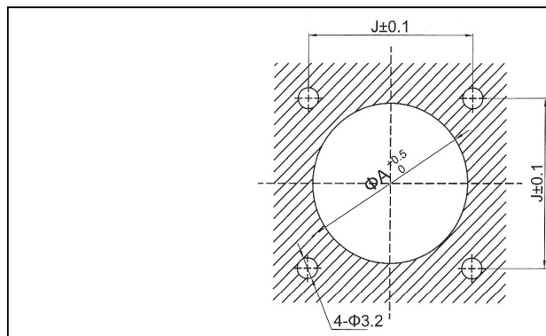
XC、XCH、XC-F-M、XCB插座面板切孔建议尺寸（前安）
