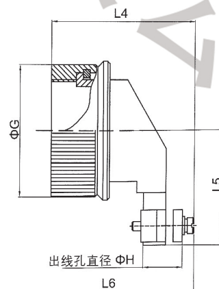
弯式电缆夹 (W)
