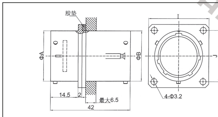
XC、XCH、XC-F-M、XCB插座面板切孔建议尺寸（前安）
