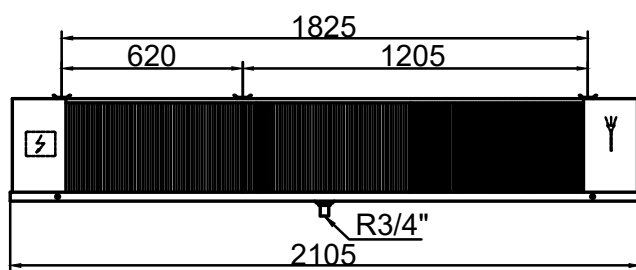
HEC/D 2503
