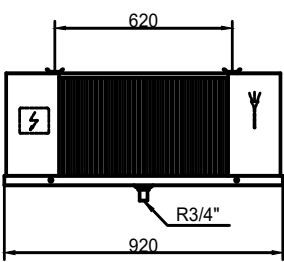
HEC/D 3001
